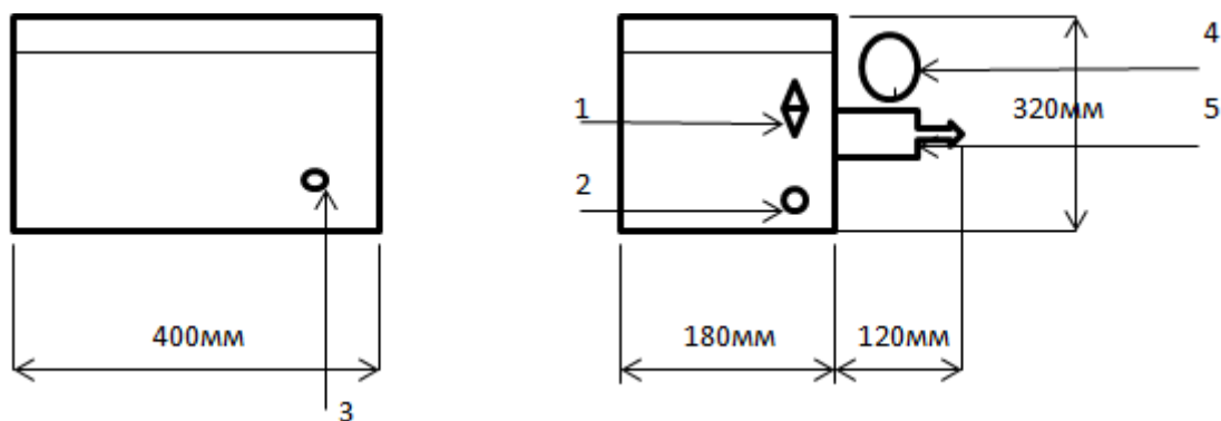
Рис.1. Устройство и размеры насоса.
